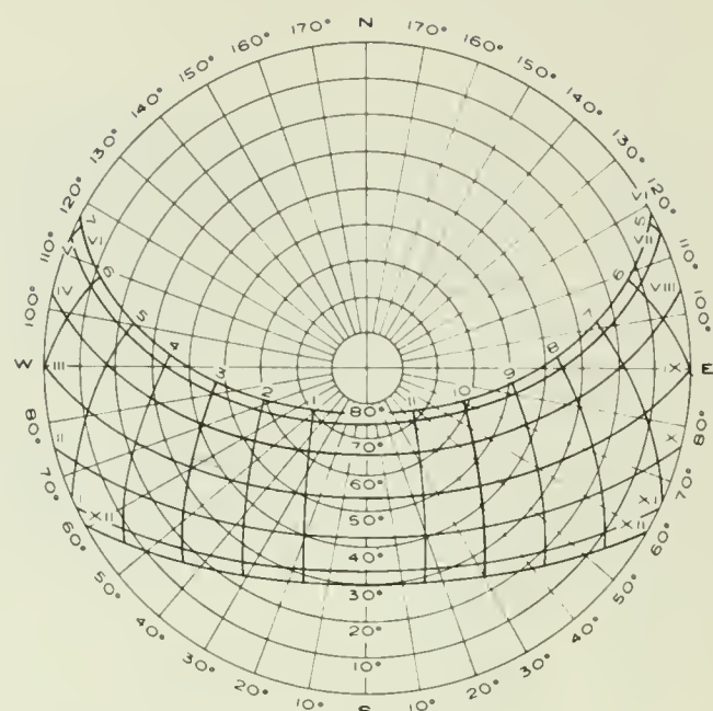
36°N LATITUDE
