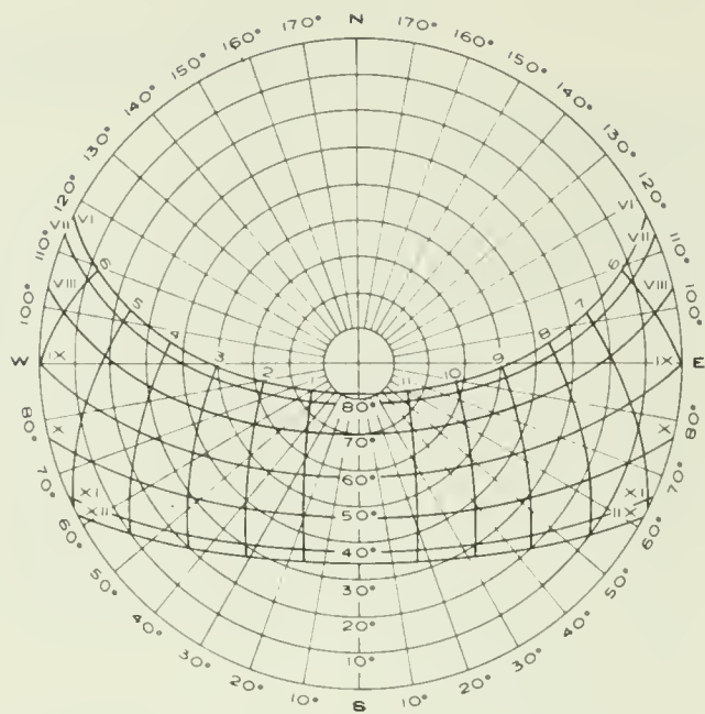
32°N LATITUDE
