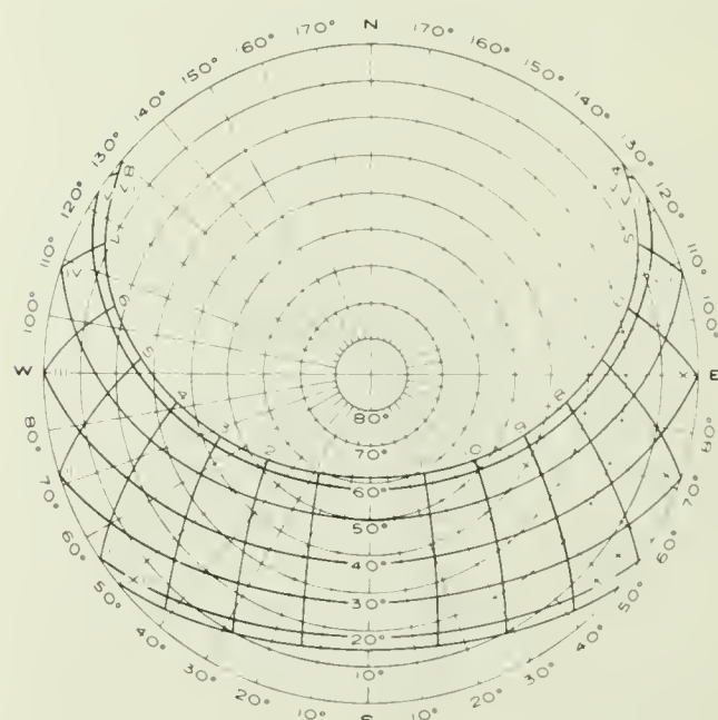
52°N LATITUDE
