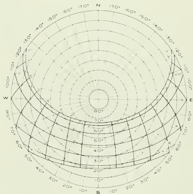
48°N LATITUDE
