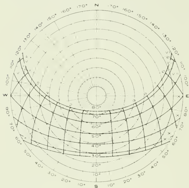
40°N LATITUDE
