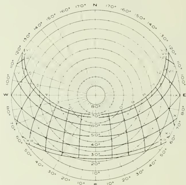
44°N LATITUDE
